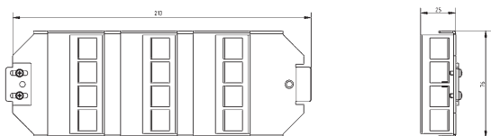
GB3 / 3x4 keystones
