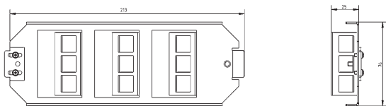
GB3 / 3x3 keystones
