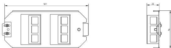
GB2 / 2x3 keystones
