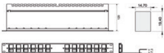
Ausschnittmaße Keystoneausbruch
